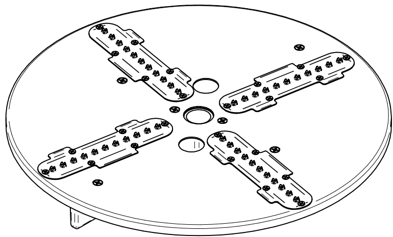
0003499 - DISCO RALADOR
