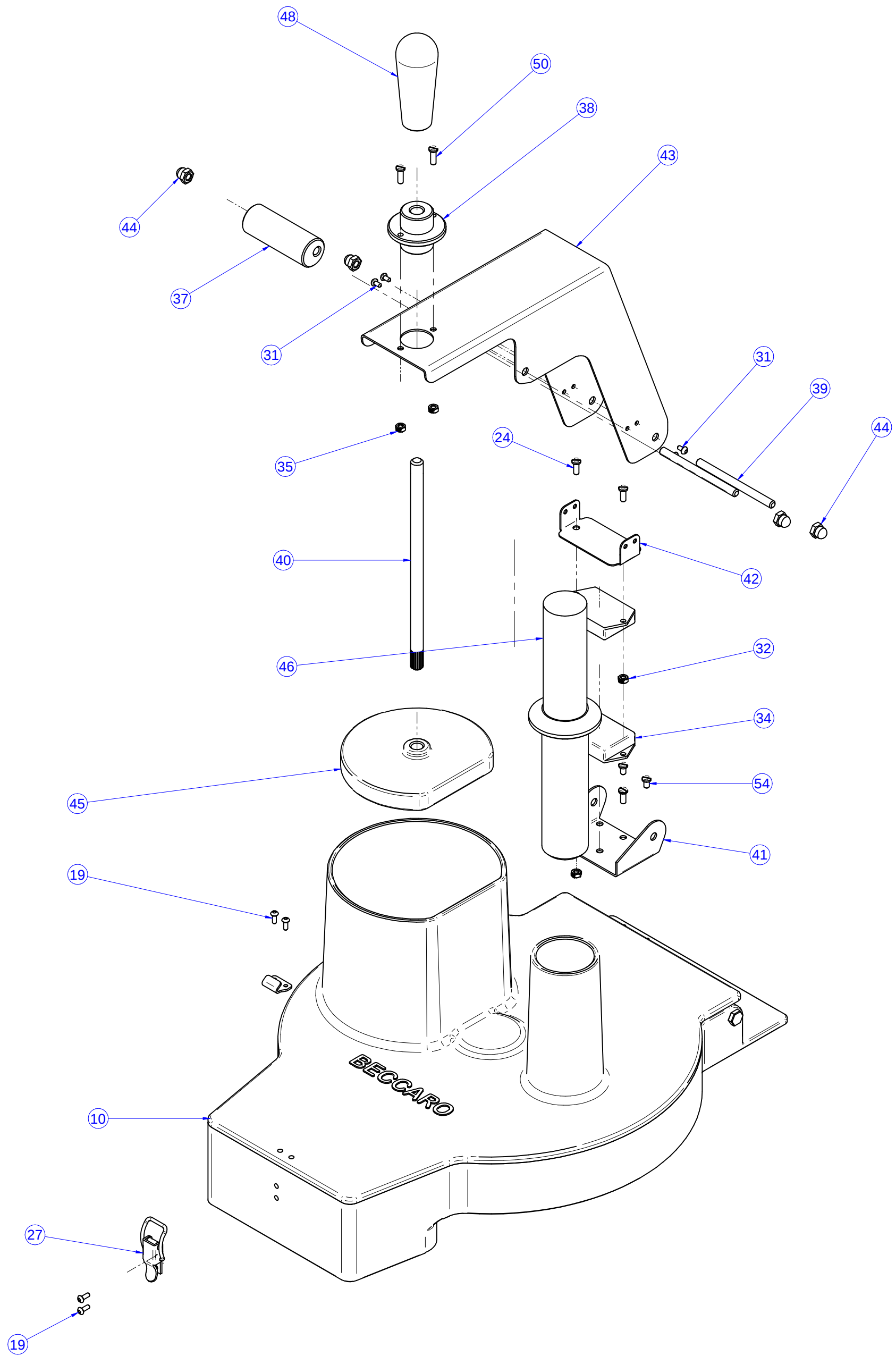
MONTAGEM DOS SUPORTES, FECHO, SENSOR E SOQUETES
