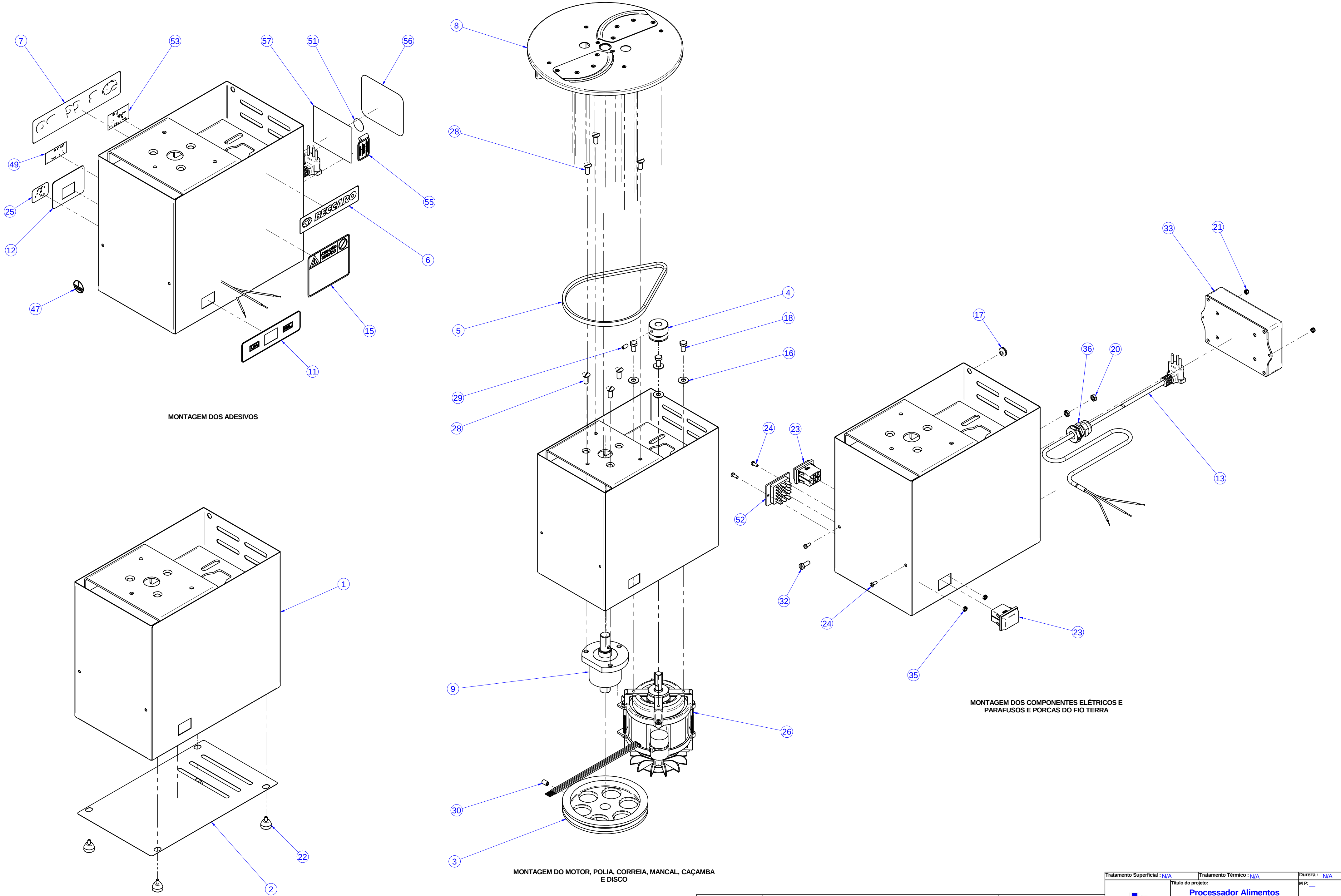
MONTAGEM DO FUNDO PROTETOR E PÉS
