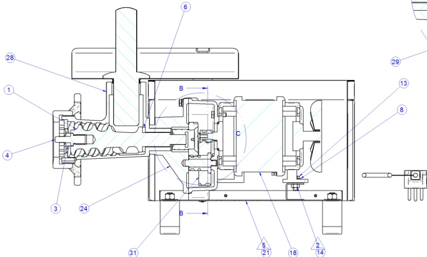
CORTE A-A
