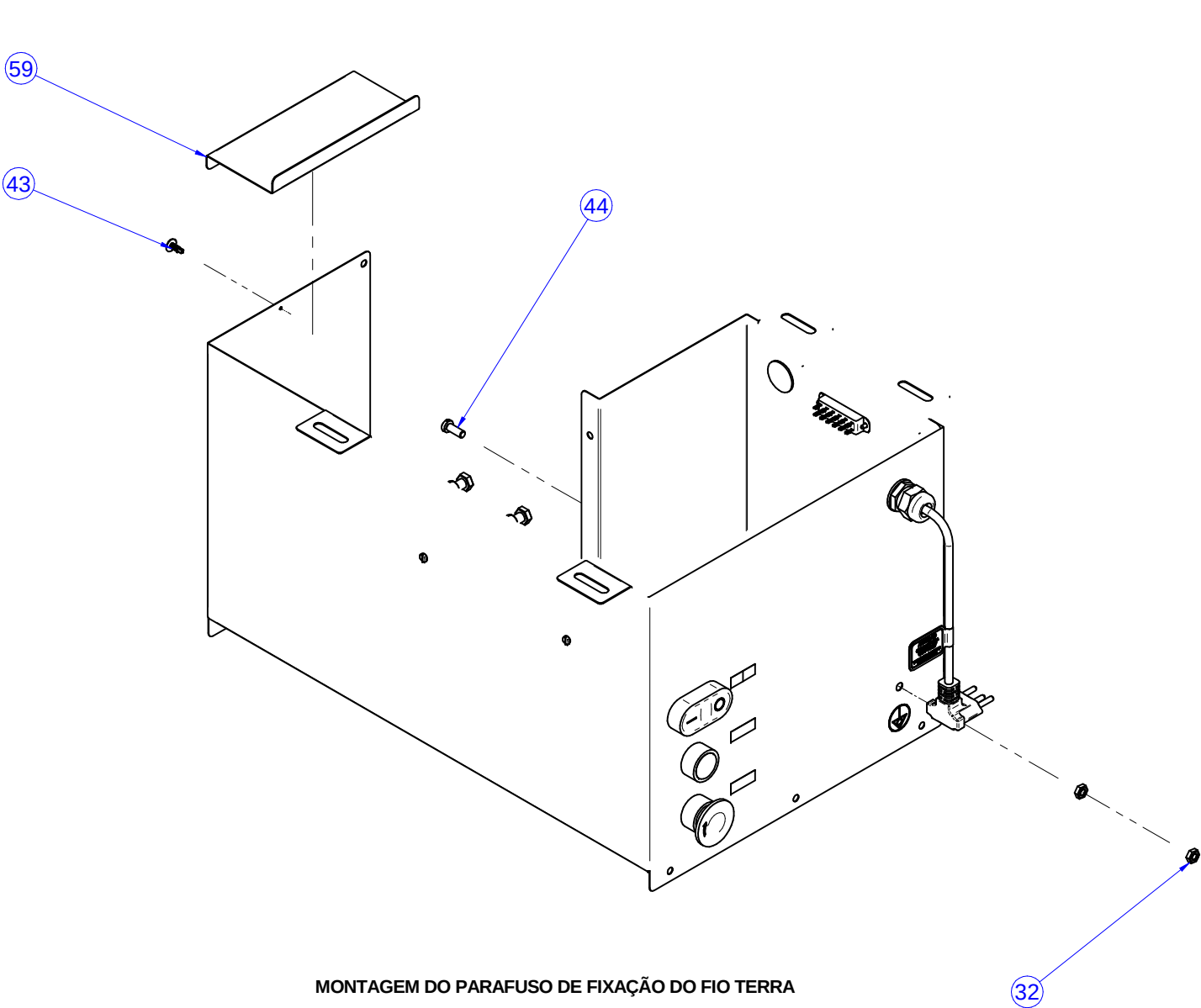
MONTAGEM DO PARAFUSO DE FIXAÇÃO DO FIO TERRA
