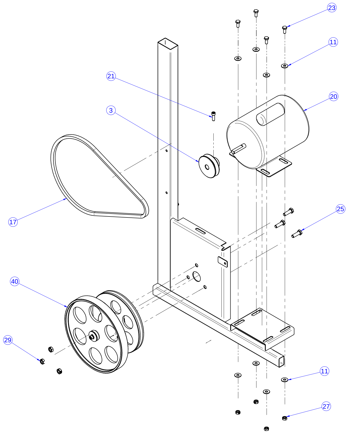
MONTAGEM DO MANCAL INFERIOR, POLIA, CORREIA E MOTOR
