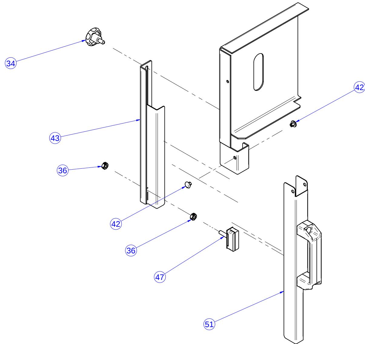
MONTAGEM DO CORPO PROTETOR, GUIA E TACO COMPLETO DA LÂMINA
