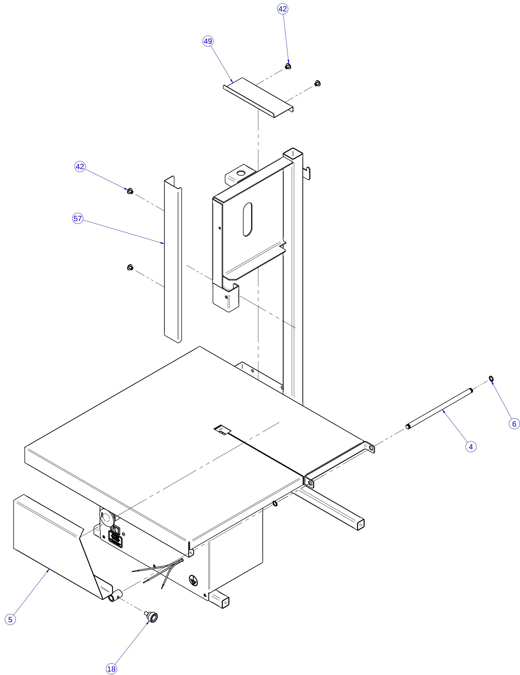
MONTAGEM DO PROTETOR DA COLUNA, FIXAÇÃO DO REGUALADOR DE BIFE E ACABAMENTO SUPERIOR DO GABINETE
