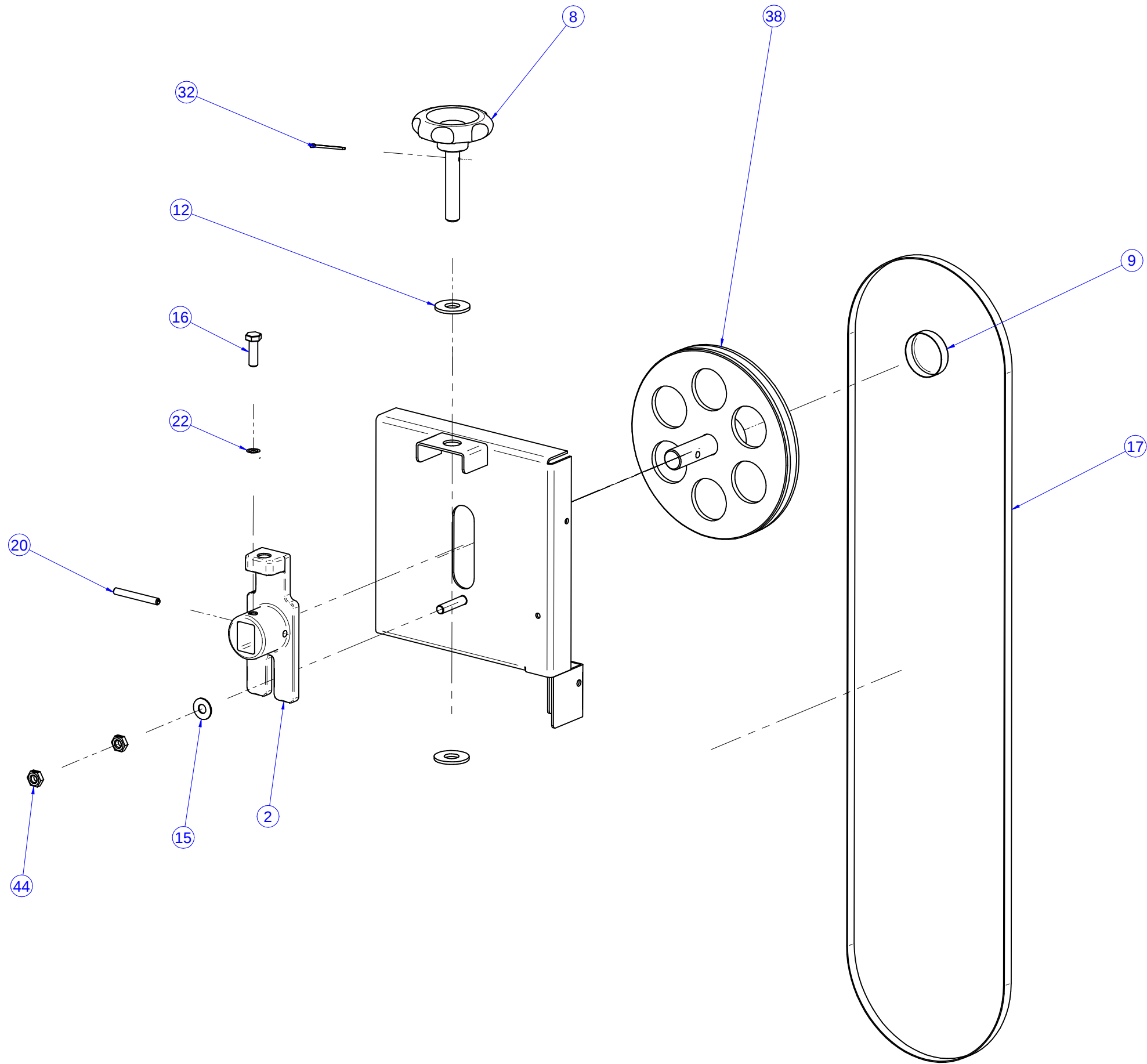
MONTAGEM DA LÂMINA, ESTICADOR , MANÍPULO, VOLANTE SUPERIOR E PROTETOR DO ROLAMENTO
