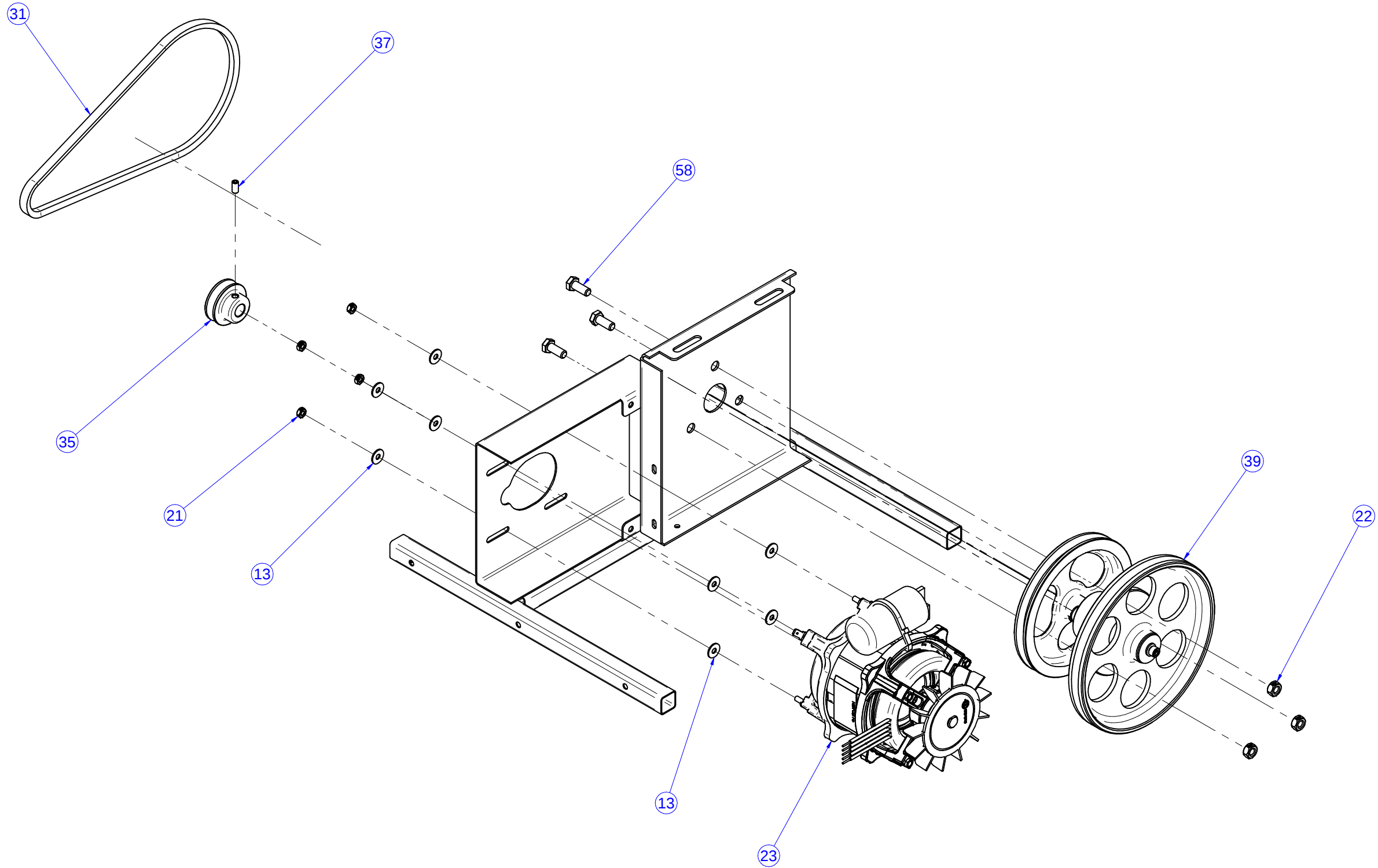
MONTAGEM DO MOTOR, POLIA, CORREIA E MANCAL COMPLETO
