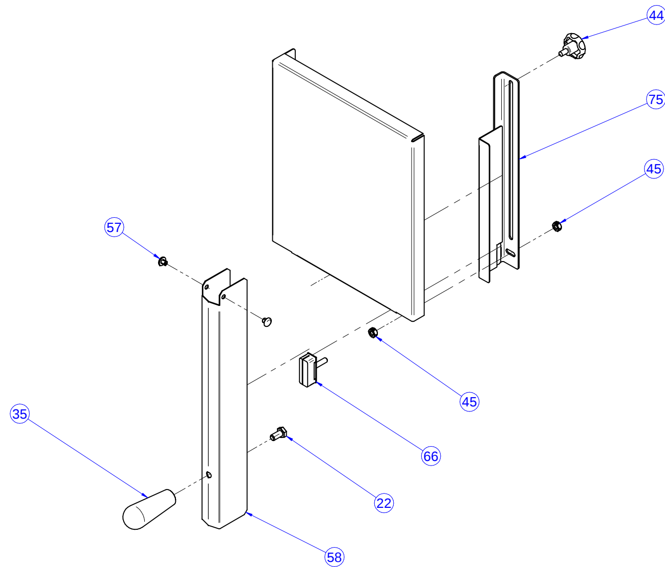
MONTAGEM DO GUIA DA LÂMINA, TACO DO GUIA DA LÂMINA E PROTETOR DA LÂMINA
