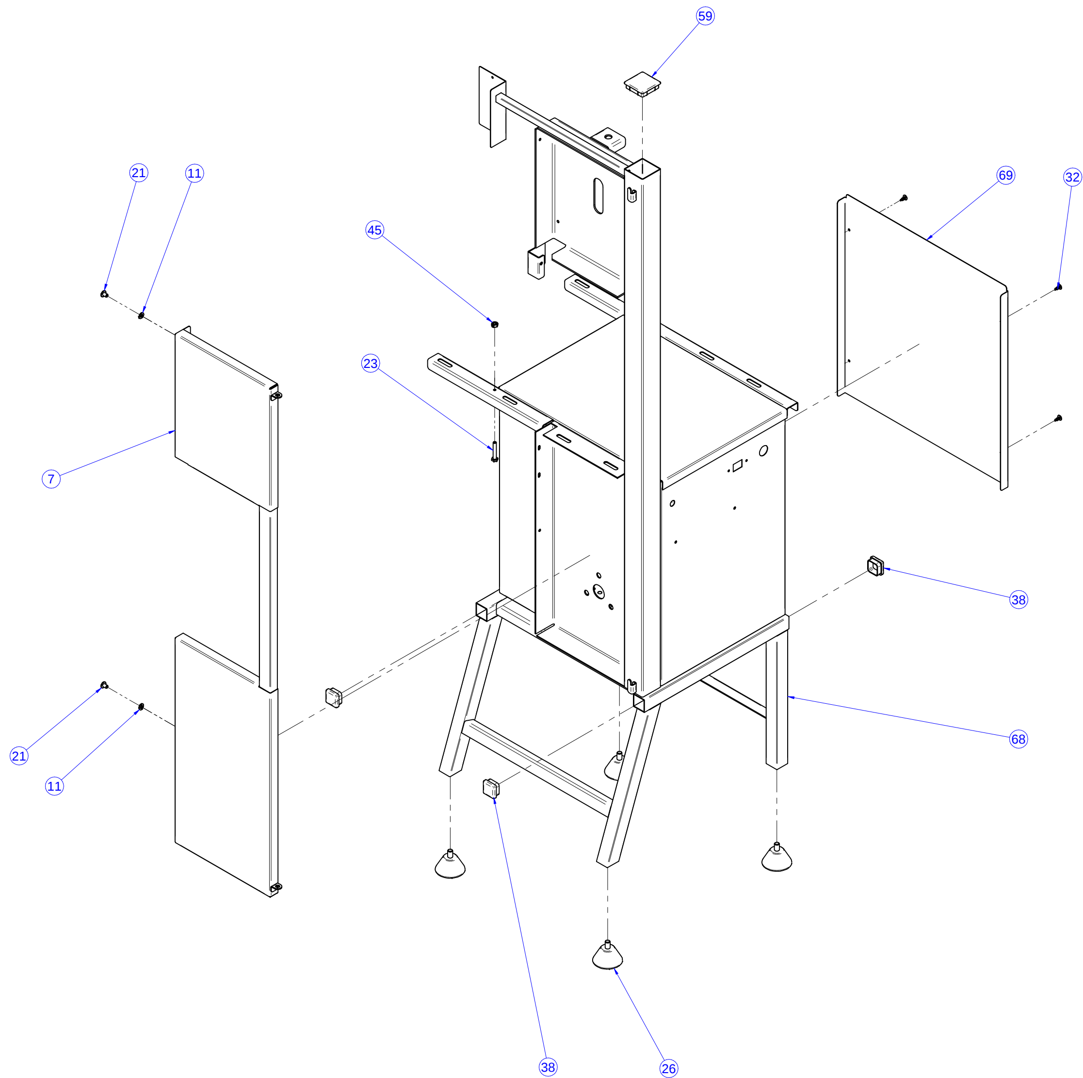
MONTAGEM DA PORTA, TRAVA DA PORTA, TAMPA TRASEIRA E PÉS DO GABINETE, BATOQUES E PARAFUSO DE BATENTE DA MESA MÓVEL
