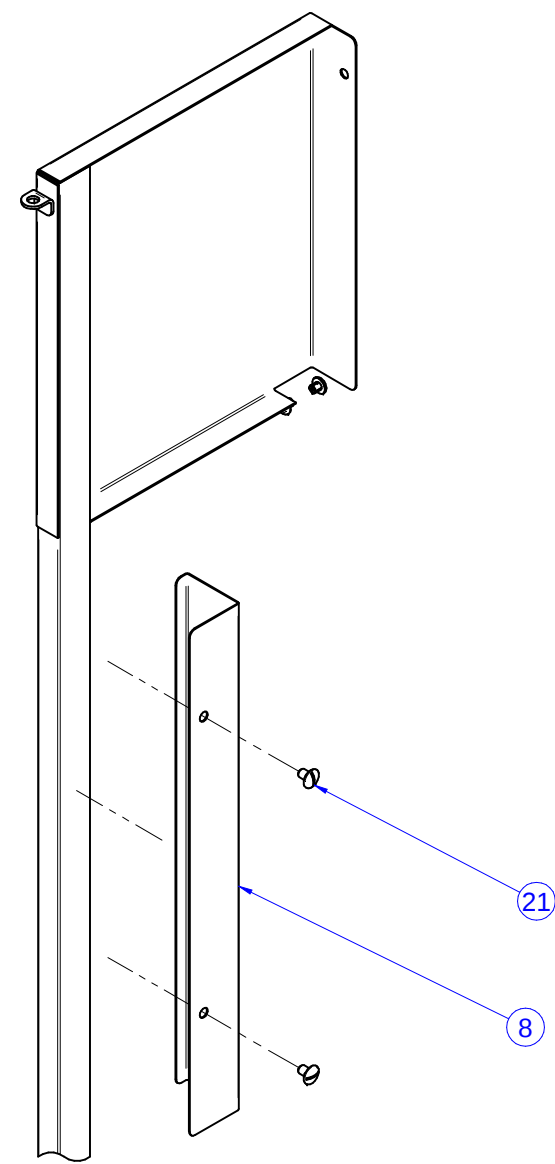
MONTAGEM DO PROTETOR DA COLUNA
