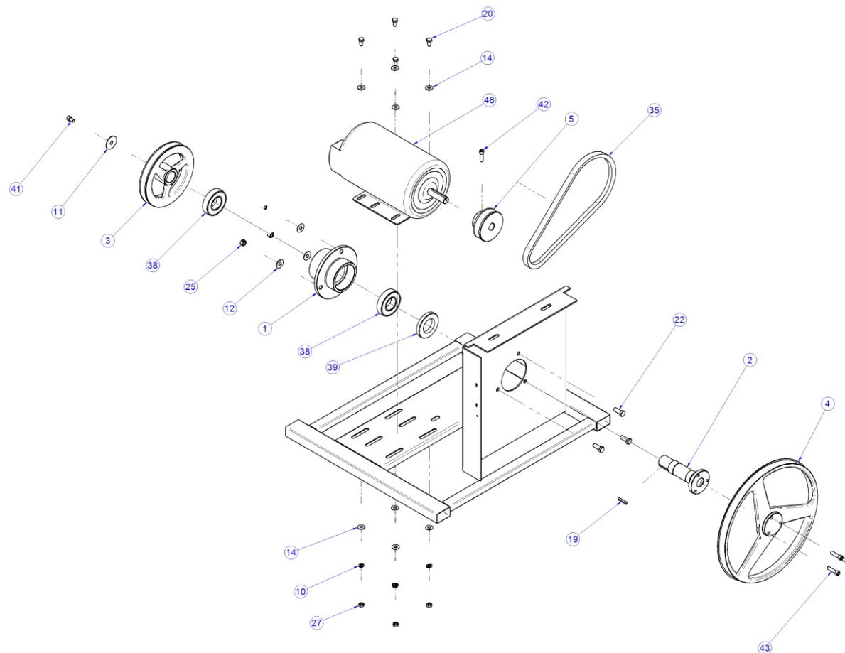
MONTAGEM DO MOTOR, POLIA, C.J. MANCAL E VOLANTE INFERIOR
