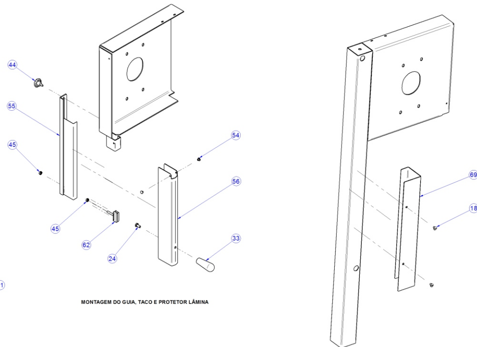
MONTAGEM DO PROTETOR COLUNA
