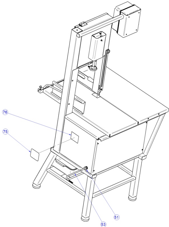
VISTA ISOMÉTRICAS
