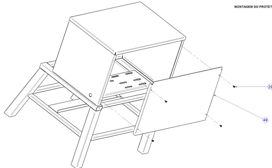
MONTAGEM TAMPA TRASEIRA
