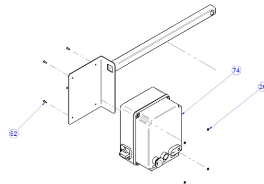
MONTAGEM DA CAIXA DE COMPONENTES ELÉTRICOS
