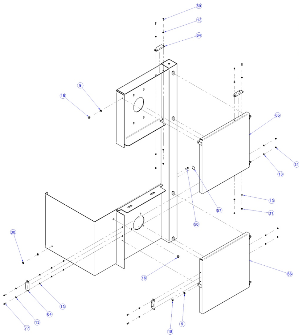
MONTAGEM DAS PORTAS, PARAFUSOS PORCAS FIO TERRA E SENSOR
