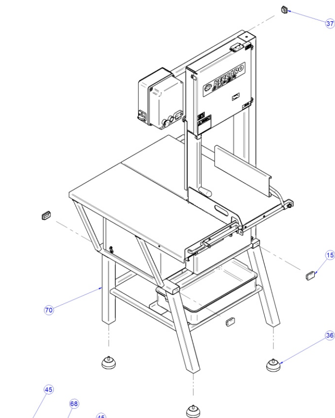
MONTAGEM DOS PÉS E BATOQUES
