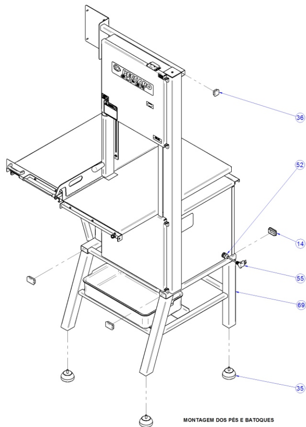
MONTAGEM DOS PÉS E BATOQUES
