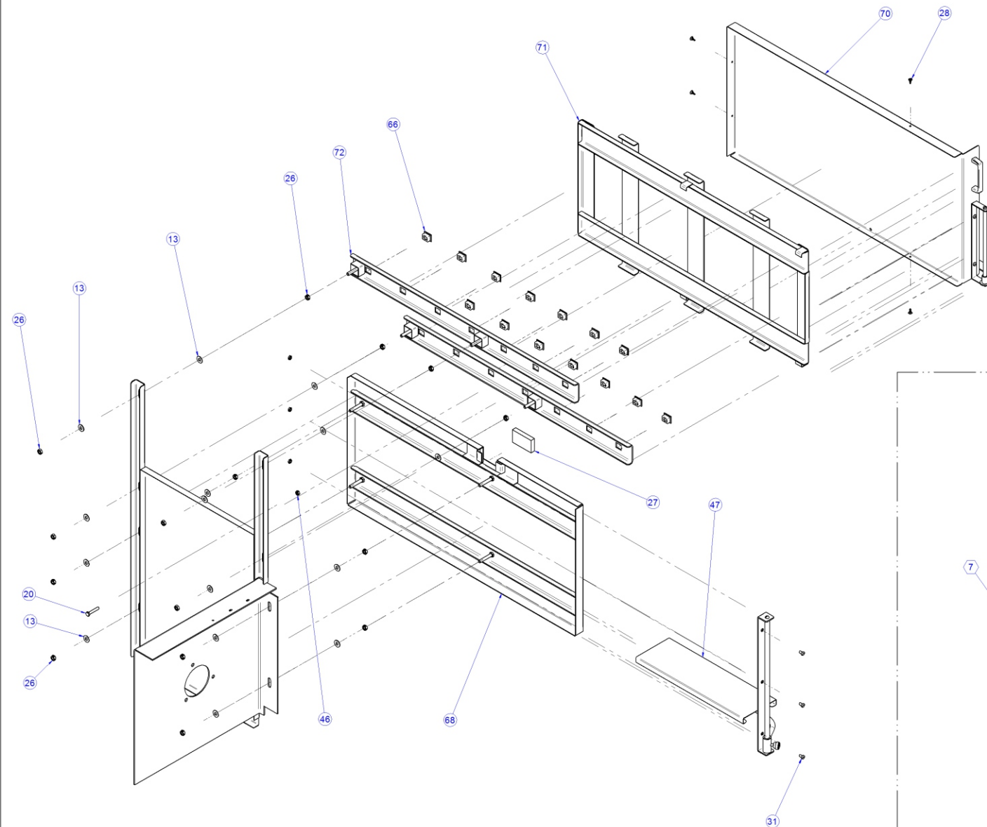
MONTAGEM BATENTE, TRILHO, SUPORTE , MESA MÓVEL, REGULADOR DE BIFE E MESA FIXA
