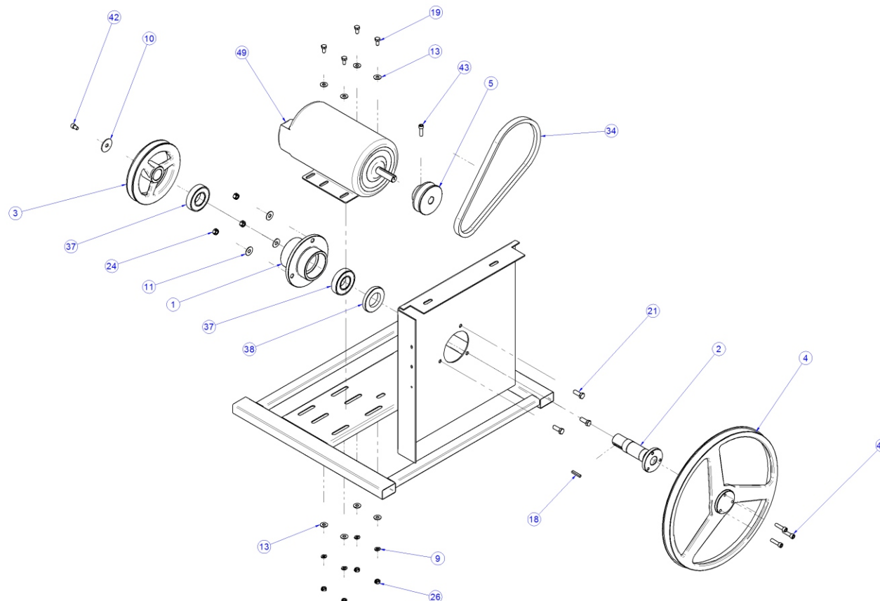
MONTAGEM DO MOTOR E MANCAL INFERIOR
