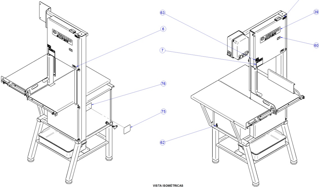
VISTA ISOMÉTRICAS
