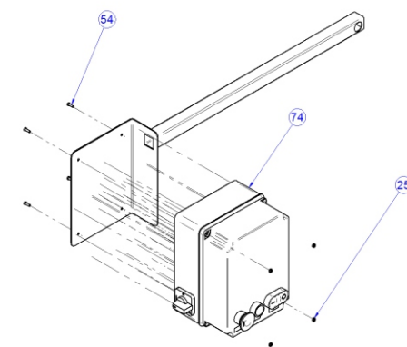
MONTAGEM DA CAIXA COMPONENTES ELÉTRICOS
